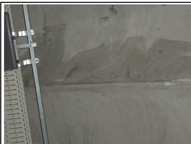
천단부 J43 조인트부 콘크리트 들뜸
